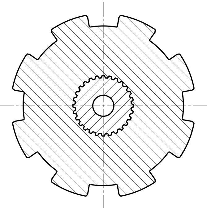
Ж-Ж (1:1) Парковочный тормоз
