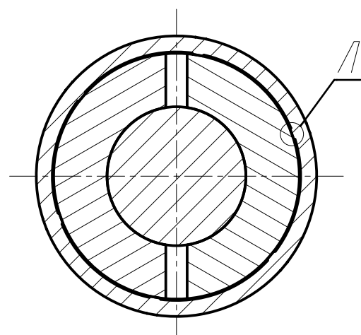
Е-Е (1:1) Установочное кольцо
